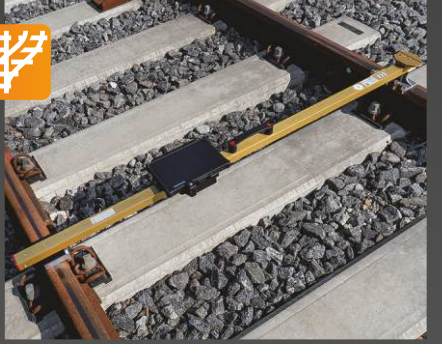
MessReg PTP II Makas muayene sistemi
